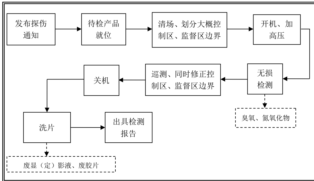
图 9-3 无损检测工作流程图
