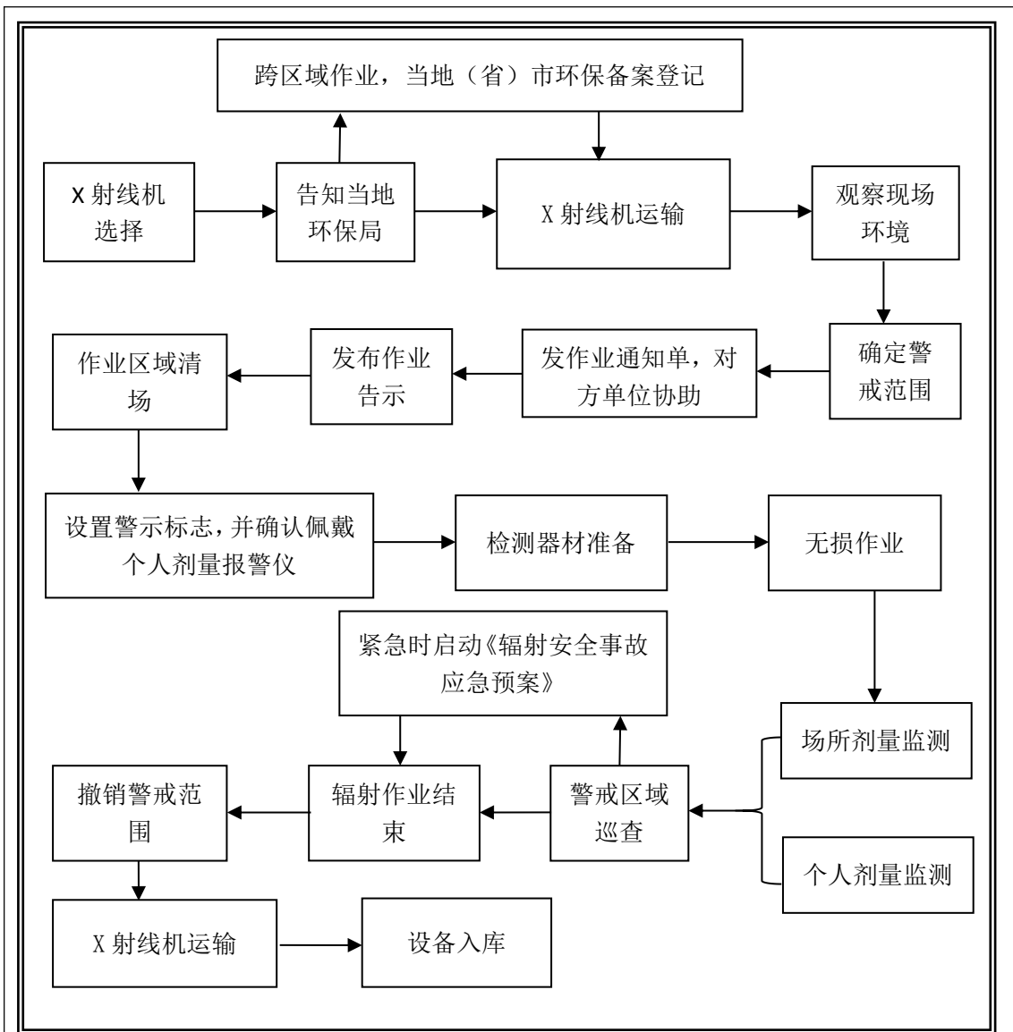
图 9-2 现场探伤工作流程图
