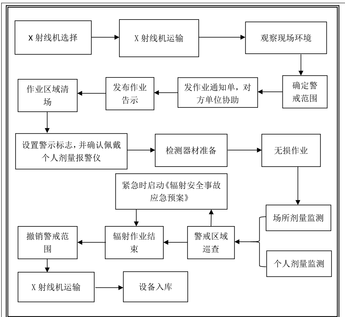
图 9-2 现场探伤工作流程图
