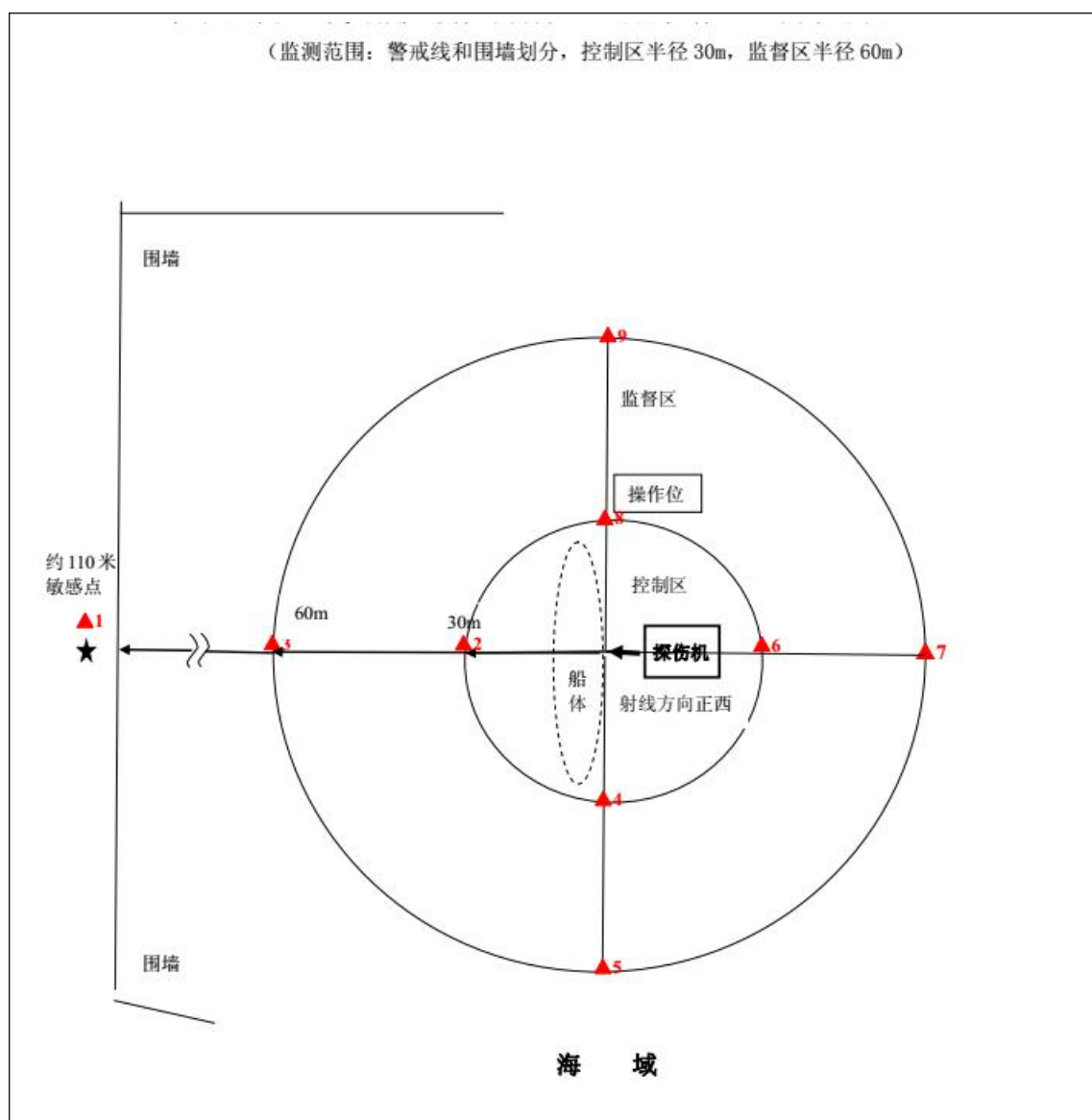
图 11-1 舟山市实诚无损检测有限公司探伤作业监测示意图
