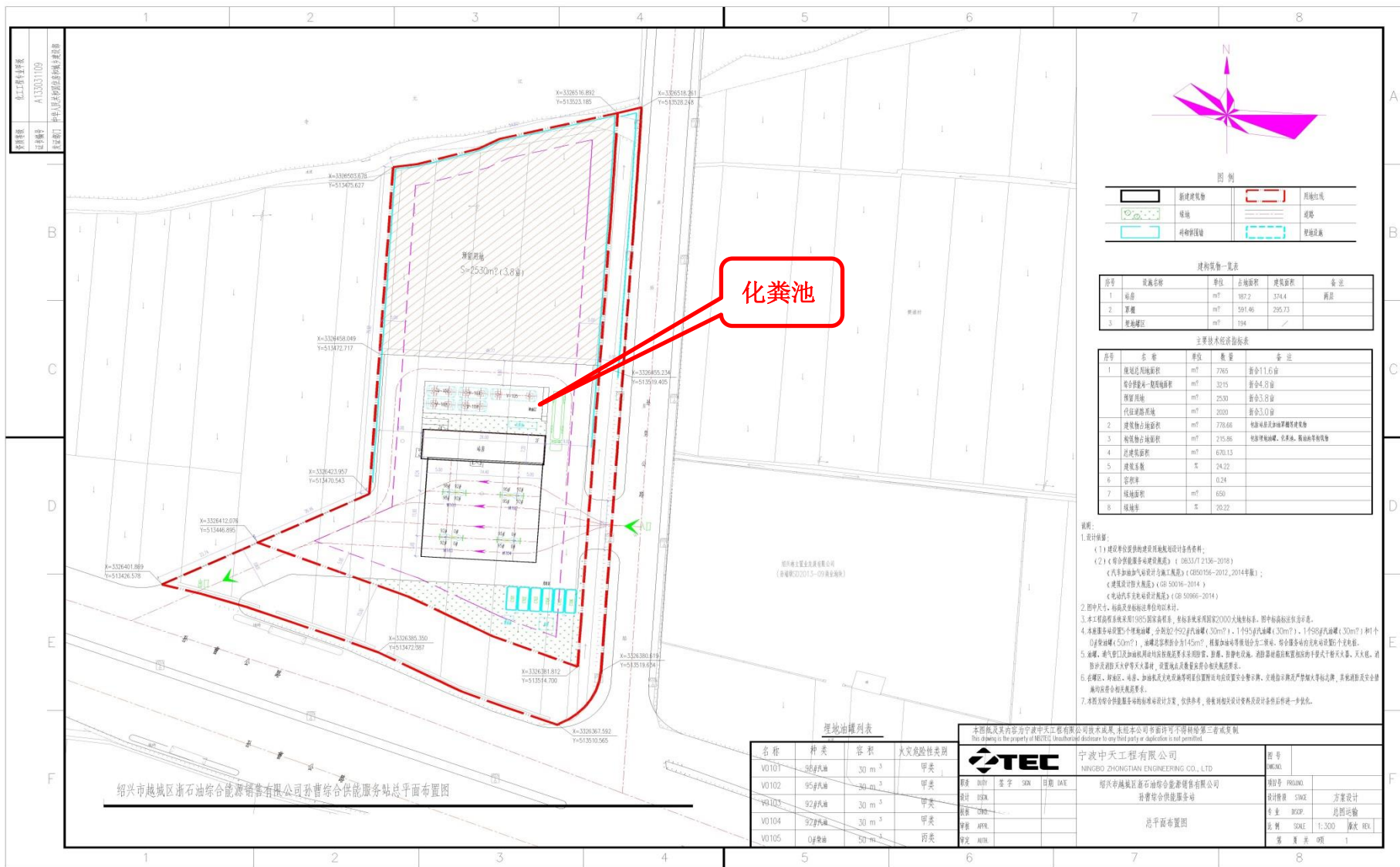
附图 3 建设项目总平面布置图
