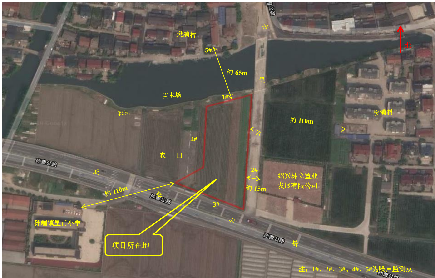
附图 2 建设项目周围环境概况及噪声监测布点图
