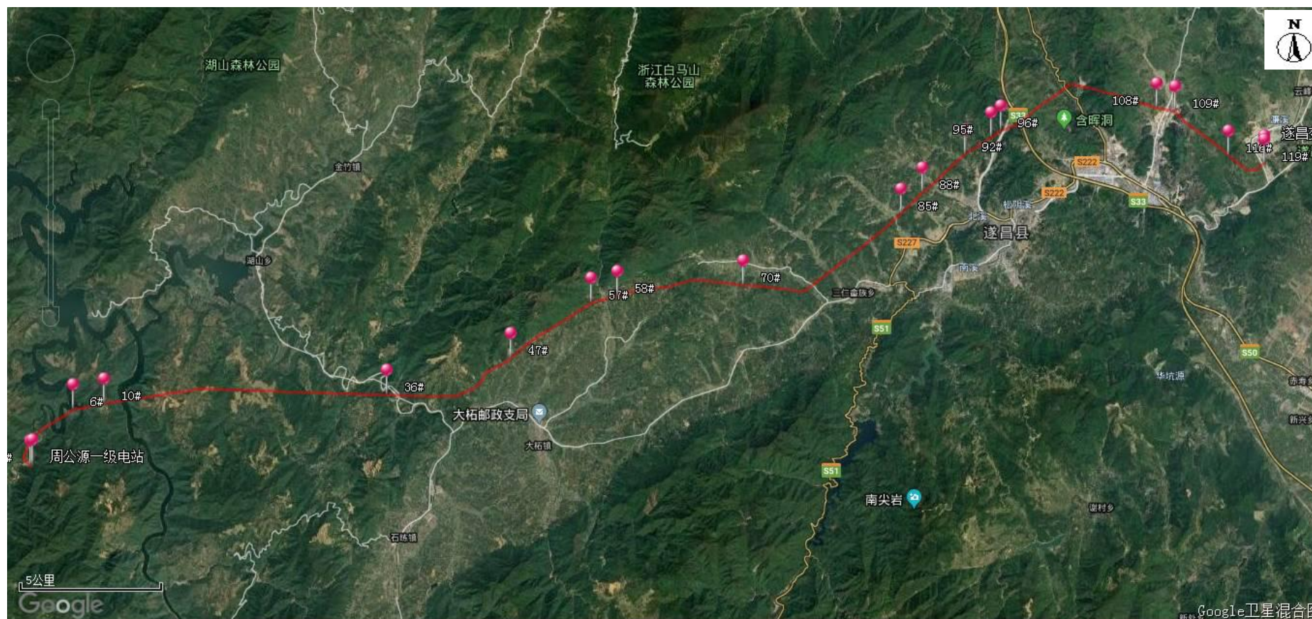
图 4-2 (2) 110kV 周遂 1242 线线路路径图
