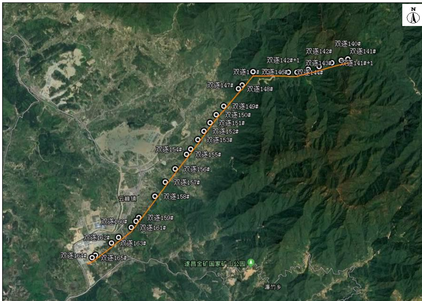
图 4-2 (1) 220kV 双遂 2389 线（丽水段）线路路径图
