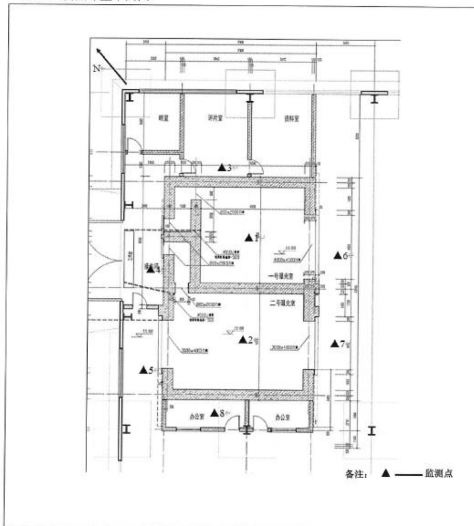
(2) 监测点布置平面图:
