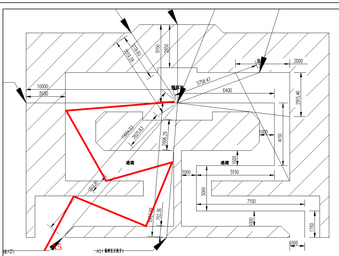
图 11-3 辐照室散射预测点位示意图
