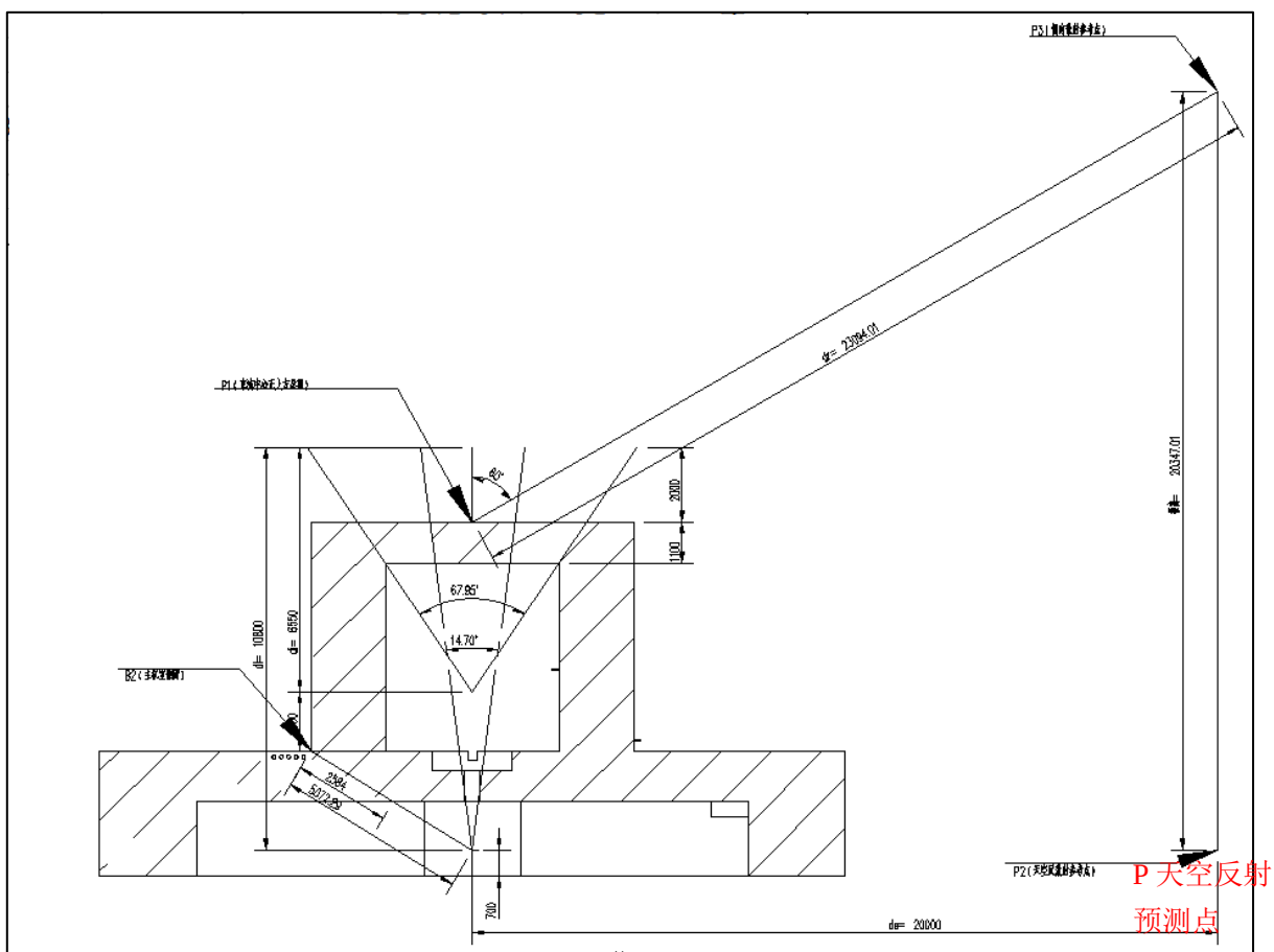
图 11-5 天空反射预测点位示意图
